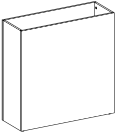
M-FCBP Planter Box W: 12"-15" D: 30"- 60" H: 42"
