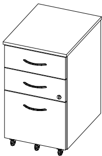
T-FPBM Mobile Box/Box/File W: 16" D: 21" H: 28"
