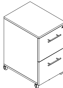
M-FPFM Mobile File/File W: 16" D: 21" H: 28"
