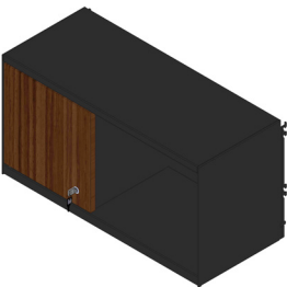
L-SPLO/ L-SPOL Split Overhead Cabinet H: 16" W: 36" - 60" D: 12"
