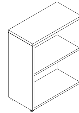
QML-SB0X Bookcase W: 24" - 42" D: 12"/15"/21" H: 29"/67"/77"
