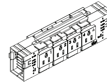
QL-EM84 Power Module
