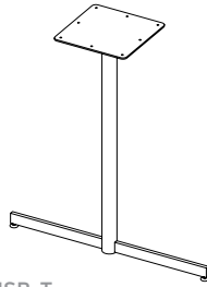
R-HSB-T Slim T-Base H: 35" D: 16"-34"
