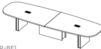
R-BE1_ Super Ellipse D: 42"-60" W: 108"-192" H: 29"
